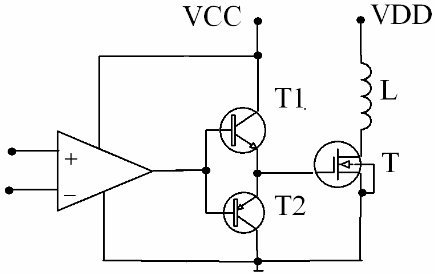
İşlemsel Kuvvetlendirici ve B sınıfı sürücü tranzistorlar ile sürme
