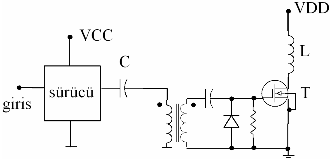
Transformatör bağışmalı sürücü
