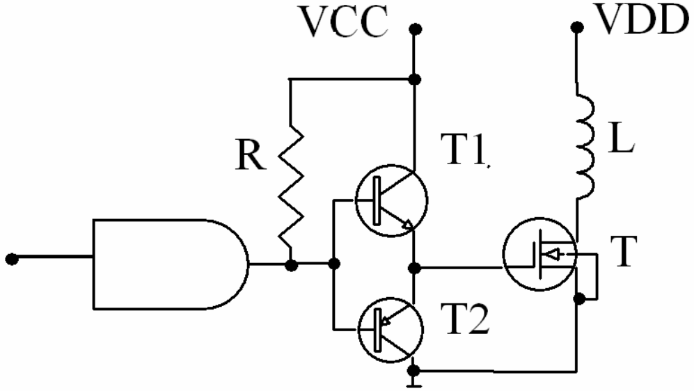
Kapı ve eşlenik tranzistorlarla sürme
