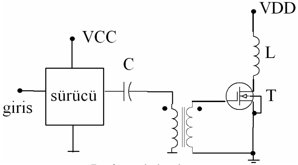
Transformatör bağışmalı sürücü
