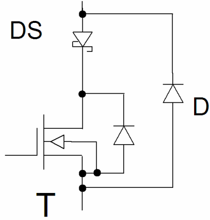
Hızlı diyotlarla koruma
