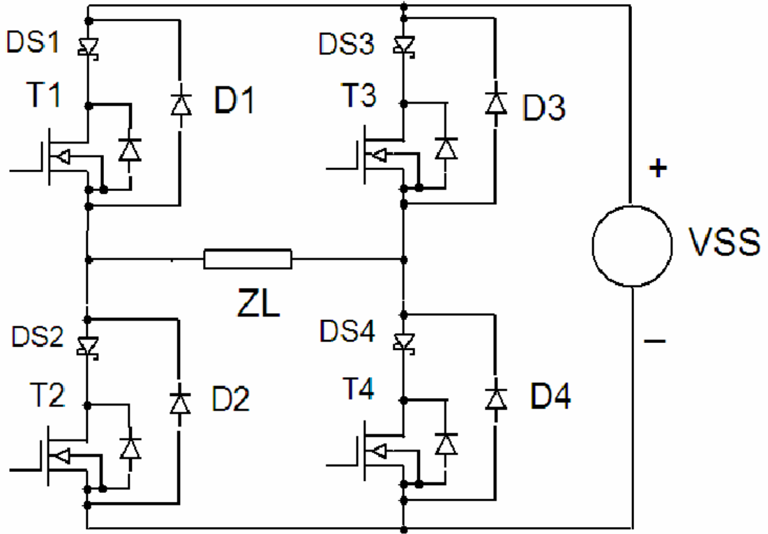
Hızlı diyotlarla korumalı köprü devresi
