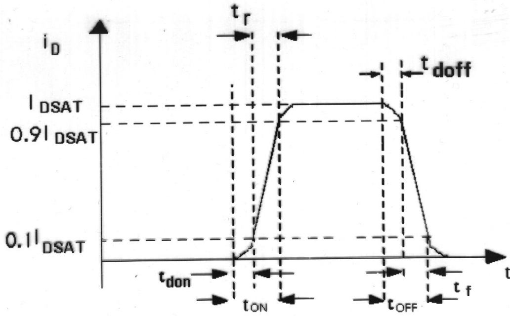
Güç MOSFET'i için anahtarlama sürelerinin tanımları
