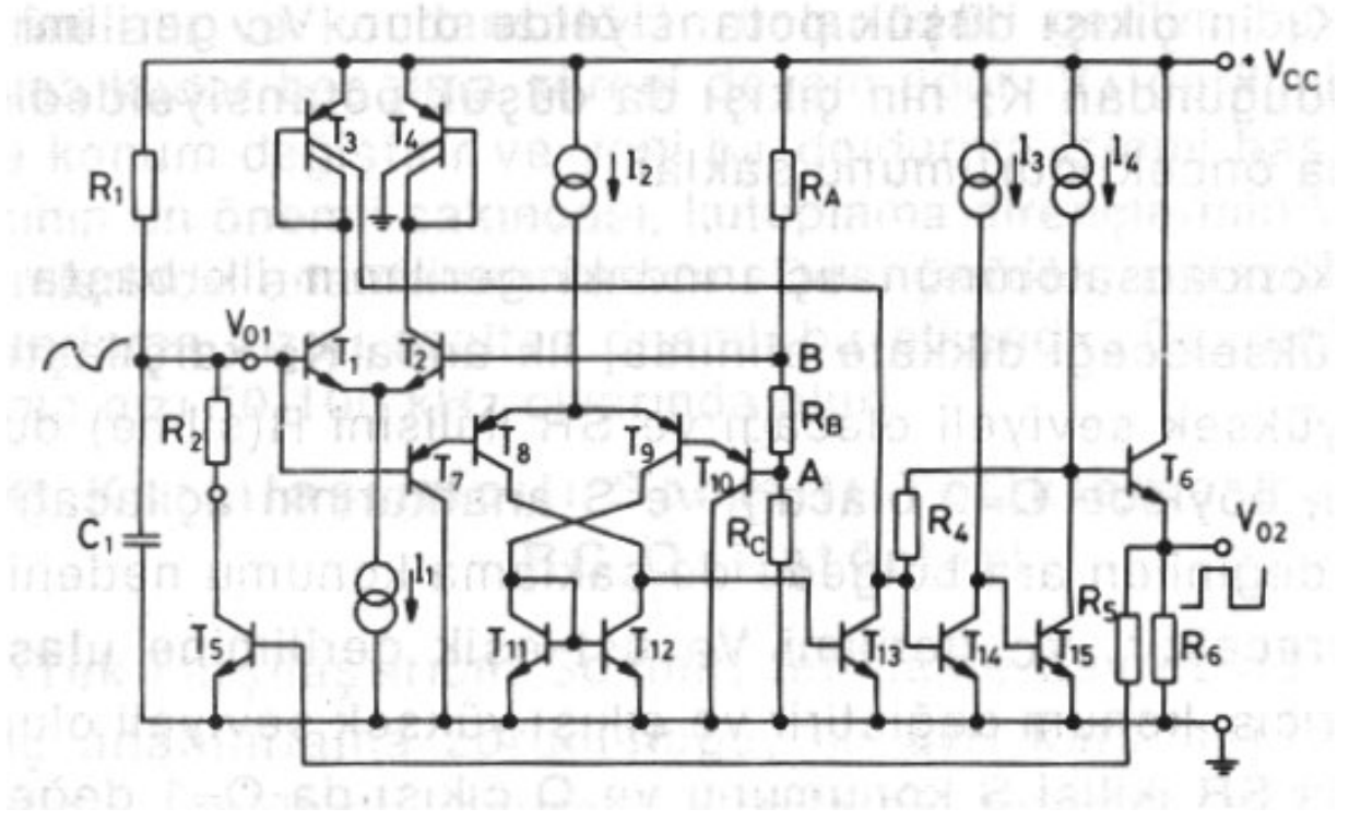
Şekil-4.7. İki karşılaştırmalı Schmitt tetikleme devresi ile kurulan RC osilatörünün tümdevre tekniği ile gerçekleştirilmesi.
