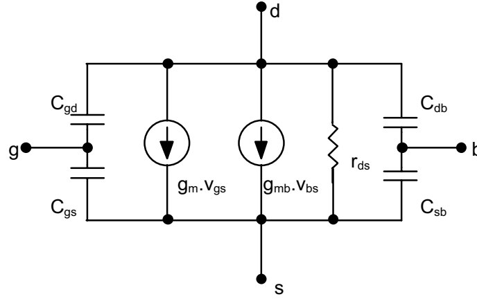
Şekil-1.2. MOS tranzistorun küçük işaret modeli
