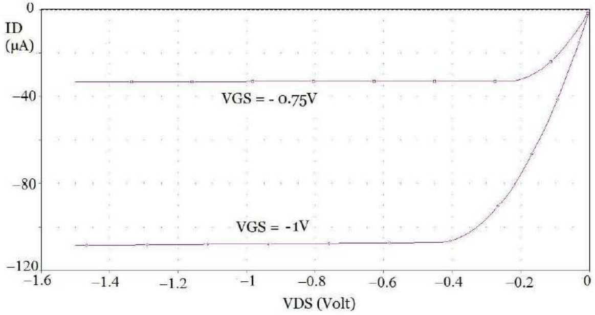
Şekil-2. PMOS transistor için çıkış özeğrileri.
