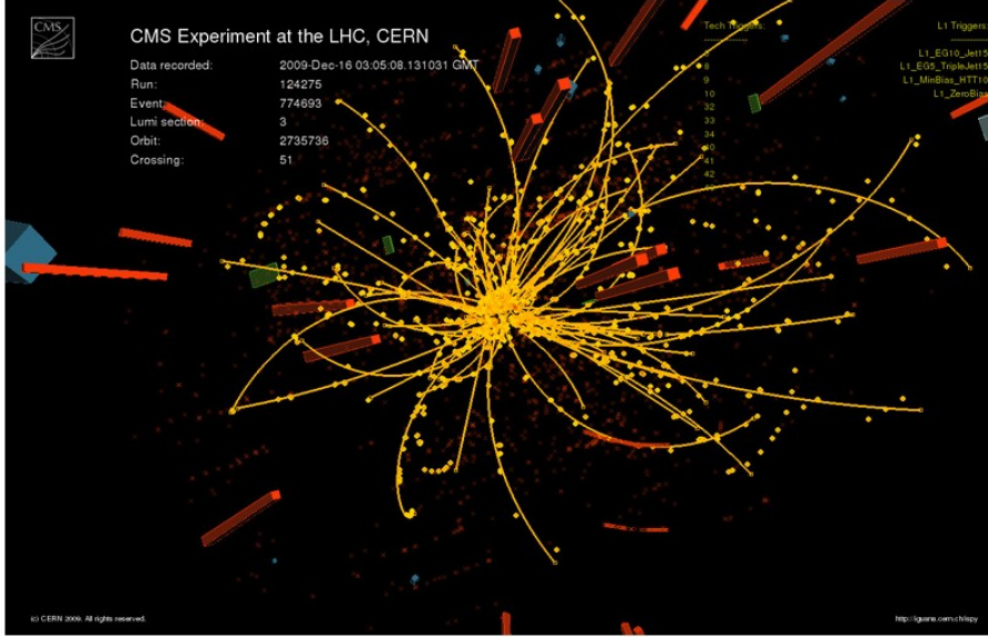
Şekil: LHC hızlandırıcısında hızlandırılan protonların CMS deneyinde çarpışması sonucu gözlemlenen olaylar
