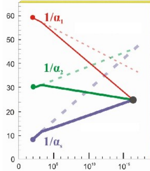
Şekil: Süpersimetri hesaba katıldığı zaman, elektromanyetik, zayıf ve yeğin (nükleer) kuvvetlerin yüksek enerjilerde birleşmesi. Noktalı çizgiler ise, Süpersimetrimin hesaba katılmadığı durumları gösterir.
