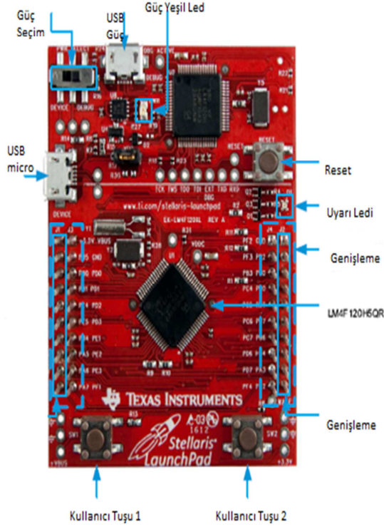
Şekil 1.4 : Geliştirme kartı.
