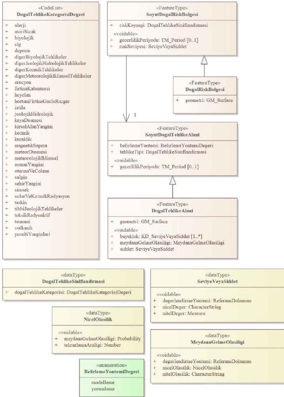
Şekil D.9 : Doğal risk bölgeleri uygulama şeması UML sınıf diyagramı.
