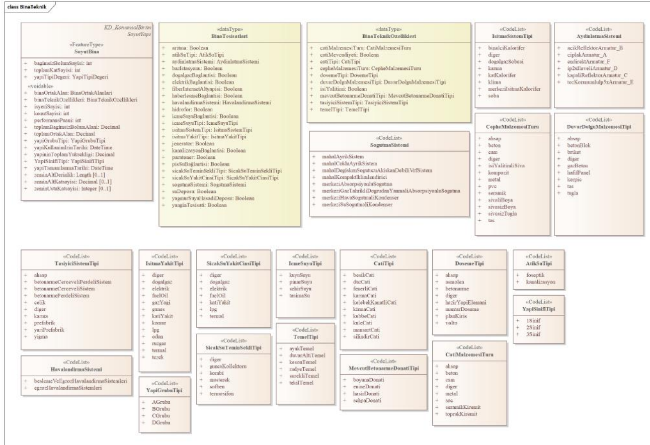
Şekil D.7 : Bina teknik uygulama şeması UML sınıf diyagramı.
