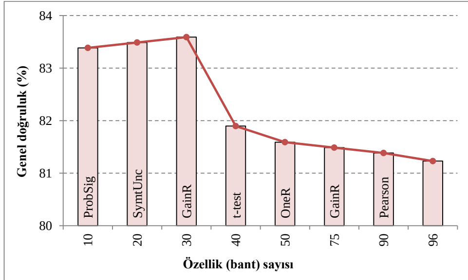
Ş ekil 6.10 : Piksel tabanlı torbalama algoritmasının özellik boyutu de ğ iř imine g ö re sınıflandırma performansı.
