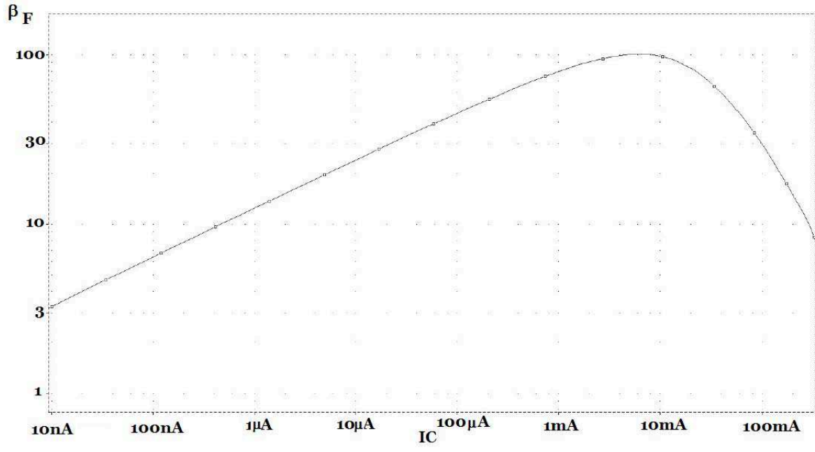
Şekil-1. \beta_F = \beta_F(I_C) değişimi. V_{BC} = 0 alınmıştır. Düşey ve yatay eksenler logaritmik olarak ölçeklenmiştir.
