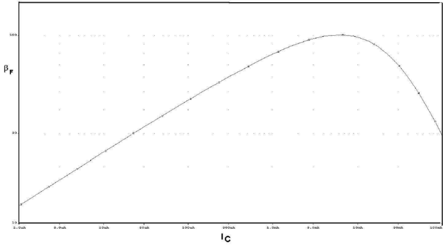
Şekil-2. \beta_F = \beta_F(I_C) değişimi, V_{BC} = 0 alınmıştır.
