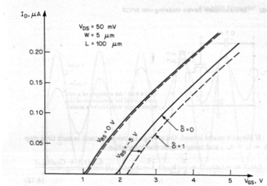
Şekil-5.20. 2. düzey modelden hesaplanan I_D akımının \delta parametresi ile değişimi (geçiş karakteristiği)
