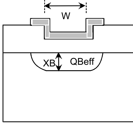
Şekil-5.19. Kanal sınırlarındaki fakirleşmiş bölgeler tarafından azaltılmış Q_B taban yükünün geometrik hesaplanması
