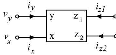
Şekil 1. DO-CCII sembolü
