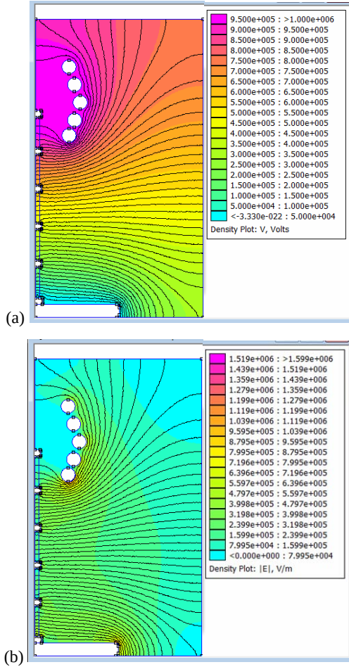
Şekil 6: Beş elektrotlu sistemde (a) potansiyel ve (b) elektrik alan dağılımı
