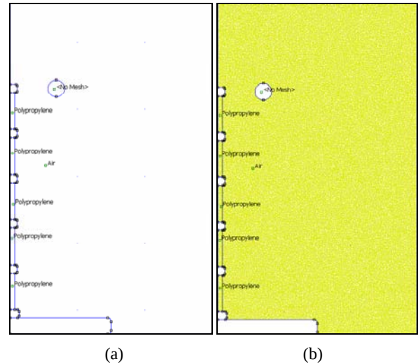
Şekil 2: Tek elektrotlu gerilim bölücü; (a) FEMM'deki çizimi; (b) Sonlu elemanlar ağı
