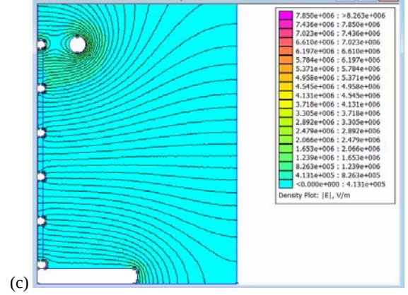
Şekil 4: Tek elektrotlu sistemde (a), (b) potansiyel ve (c) Eşpotansiyel çizgilerle birlikte elektrik alan dağılımı
