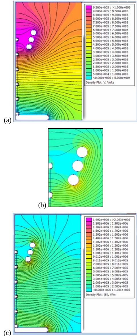
Şekil 5: Üç elektrotlu sistemde (a), (b) potansiyel ve (c) Eşpotansiyel çizgilerle birlikte elektrik alan dağılımı
