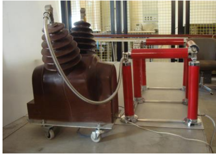
Şekil 6: Kullanılan, tekerlekli, yüksek gerilim trafosu
