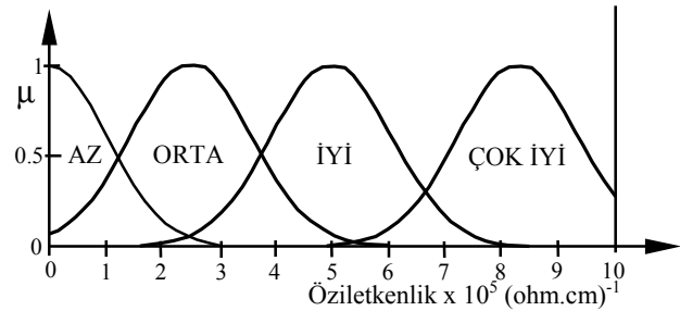
Şekil 4: iletkenlik giriş büyüklüğüne ilişkin üyelik fonksiyonları.
