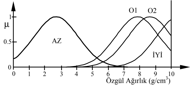
Şekil 3: Özgül ağırlık giriş büyüklüğüne ilişkin üyelik fonksiyonları.
