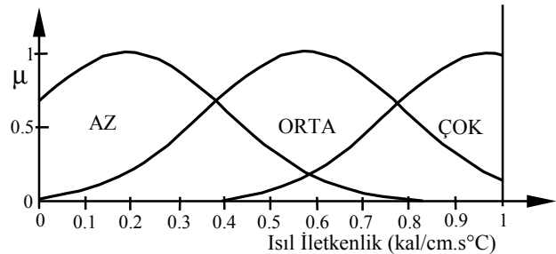
Şekil 5: Isıl iletkenlik giriş büyüklüğüne ilişkin üyelik fonksiyonları.
