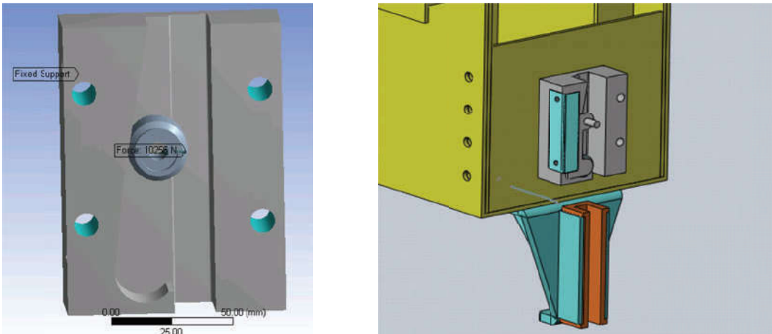
Şekil 6. Sınır şartları ve montajı
