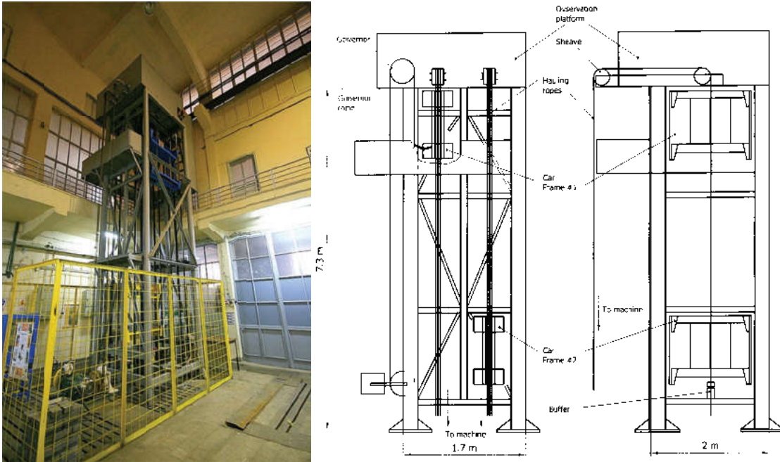
Şekil 2. İTÜ Makina Fakültesi Asansör Laboratuvarı deney test düzeneği
