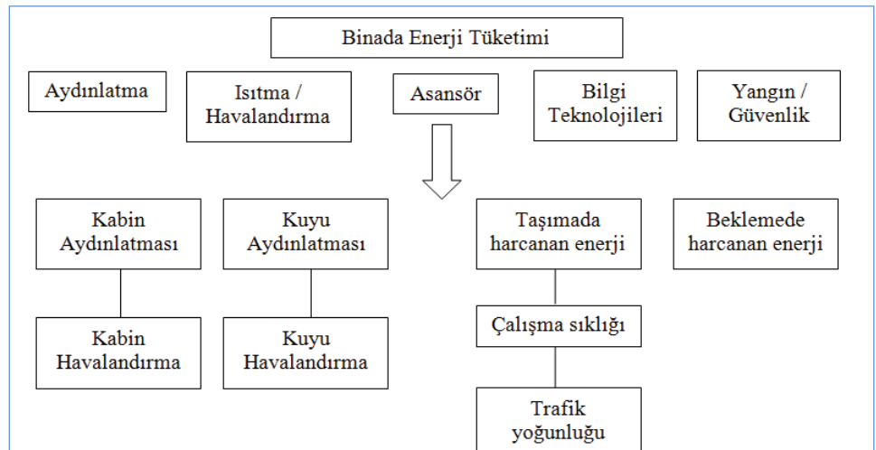
Şekil 2. Binada Enerji Tüketimi ve Asansörler
