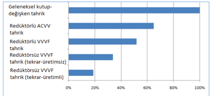
Şekil 3. Tahrik Yöntemine Bağlı Asansör Ortalama Enerji Tüketimi [3]
