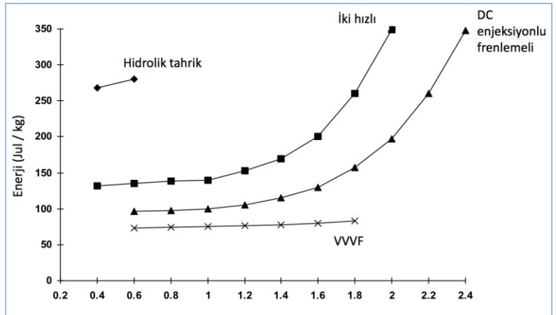
Şekil 4. Doolard Metoduna Göre Çeşitli Tipte Tahriklerde Enerji Tüketimi
