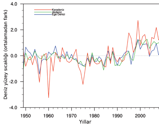
Şekil 5 Akdeniz, Ege Denizi ve Karadeniz yaz mevsimi deniz yüzey sıcaklık anomalilerinin son 60 yıldaki değişimi (°C)
