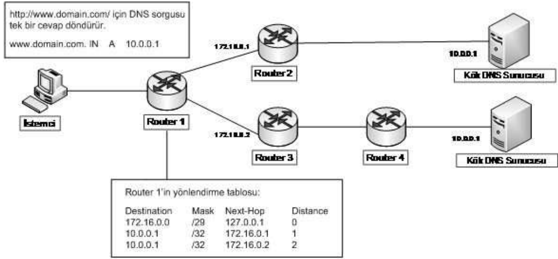
Şekil 2. Anycast çalışma yapısı
