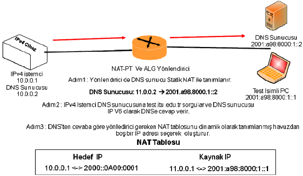
Şekil 3. IPv4 Bulutundan IPv6 Bulutuna Geçiş
