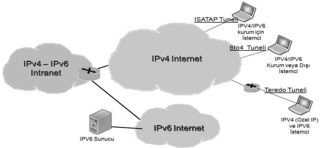
Şekil 1. Tünelleme teknikleri
