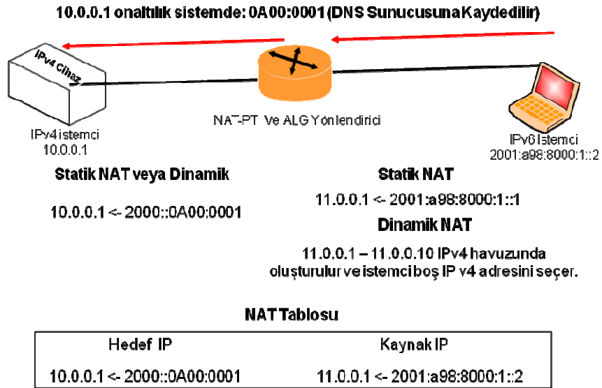
Şekil 3. IPv6 Bulutundan IPv4 Bulutuna Geçiş
