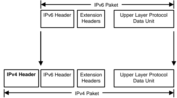
Şekil 1. IPV4 ile Kiliflanmış IPV6 Paketi
