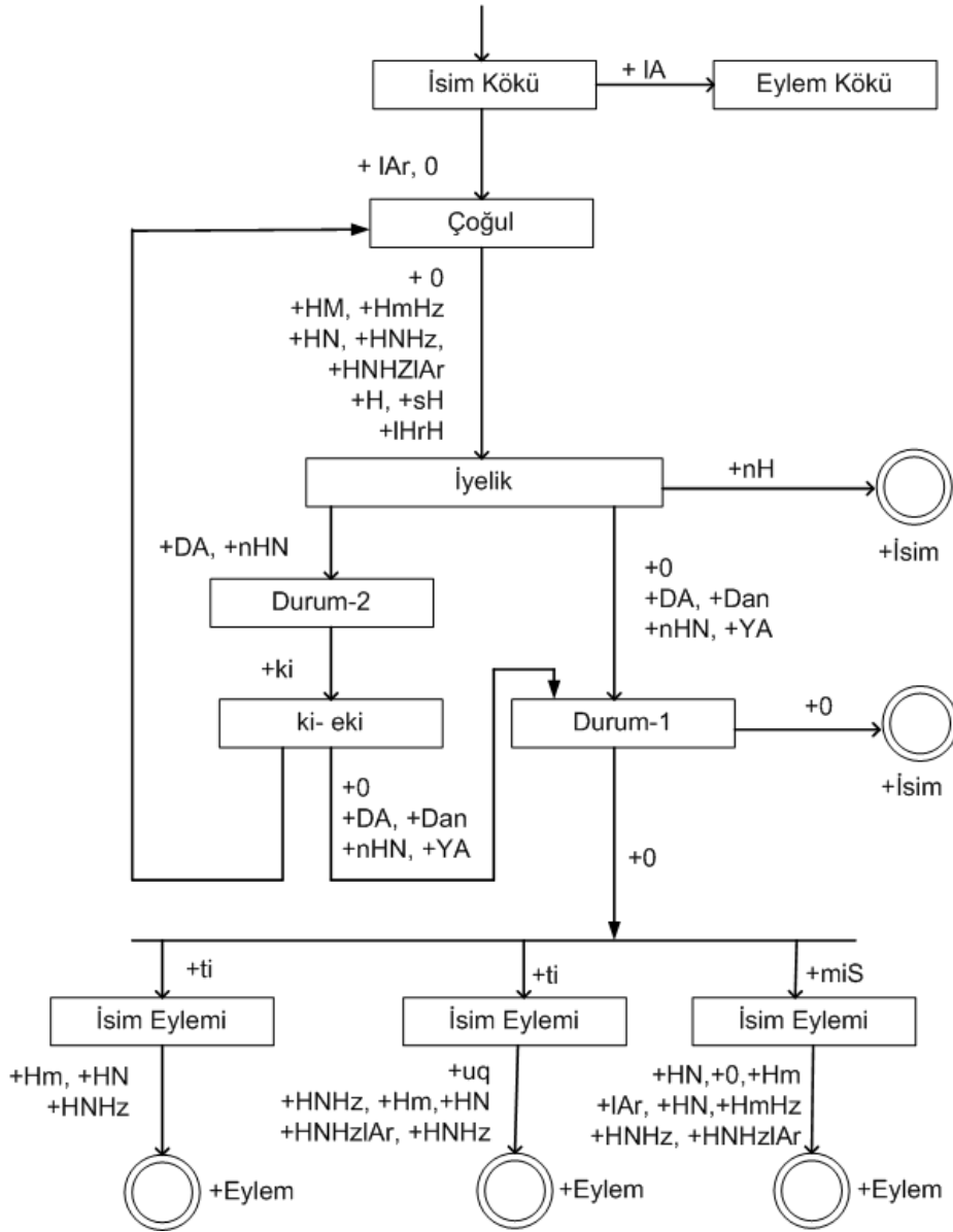
Şekil 3.7 : İsimlerin sonlu durumlu makineler ile çözümlemesi.
