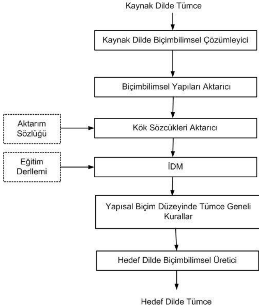
Şekil 6.2 : Karma yöntemi [55]' den uyarlanmıştır.
