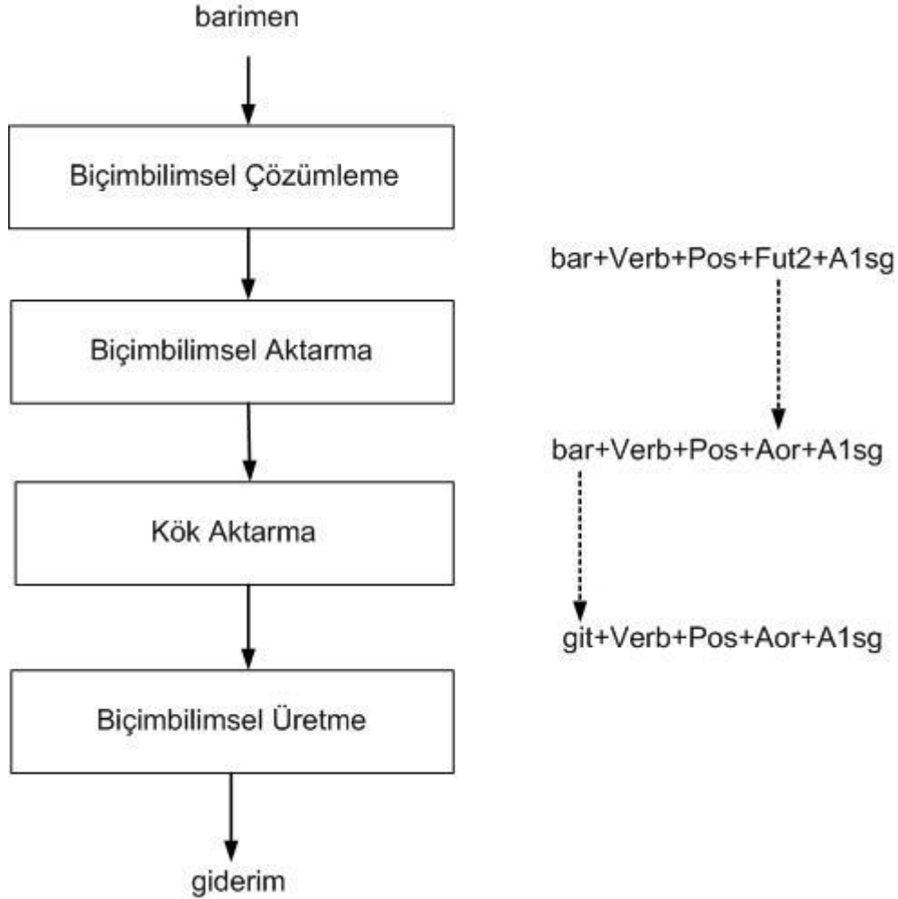
Şekil 6.1 : Uygurca sözcüğün Türkçe karşılığının doğrudan oluşturulması 20 .
