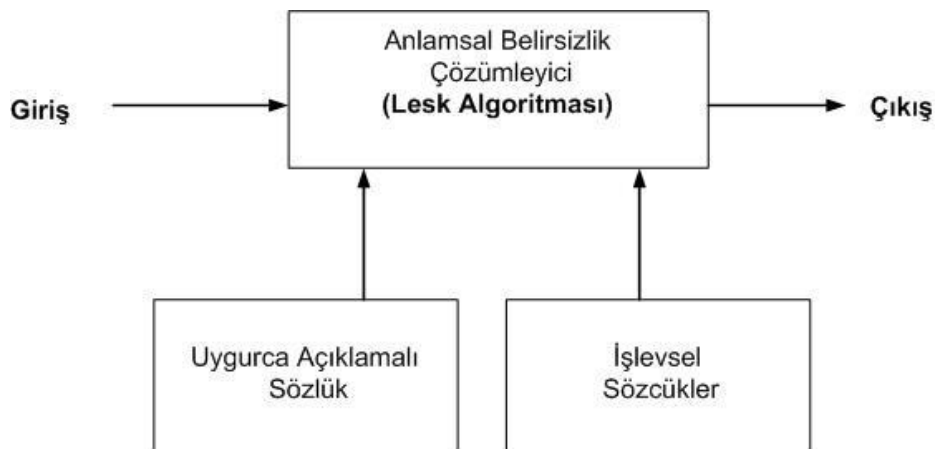
Şekil 5.4 : Anlamsal belirsizlik giderici.
