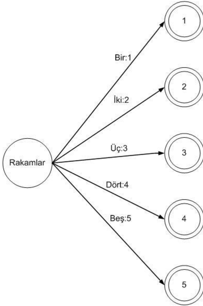
Şekil 2.4 : Sonlu durumlu dönüştürücüler.
