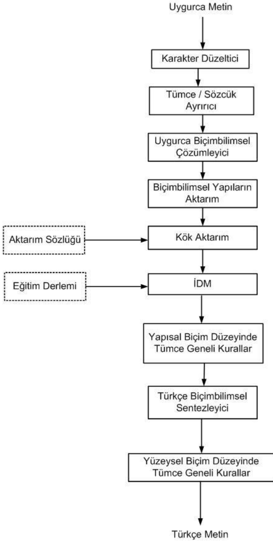
Şekil 7.1 : Karma model ile Uygurcadan Türkçeye çeviri sistemi[55]
