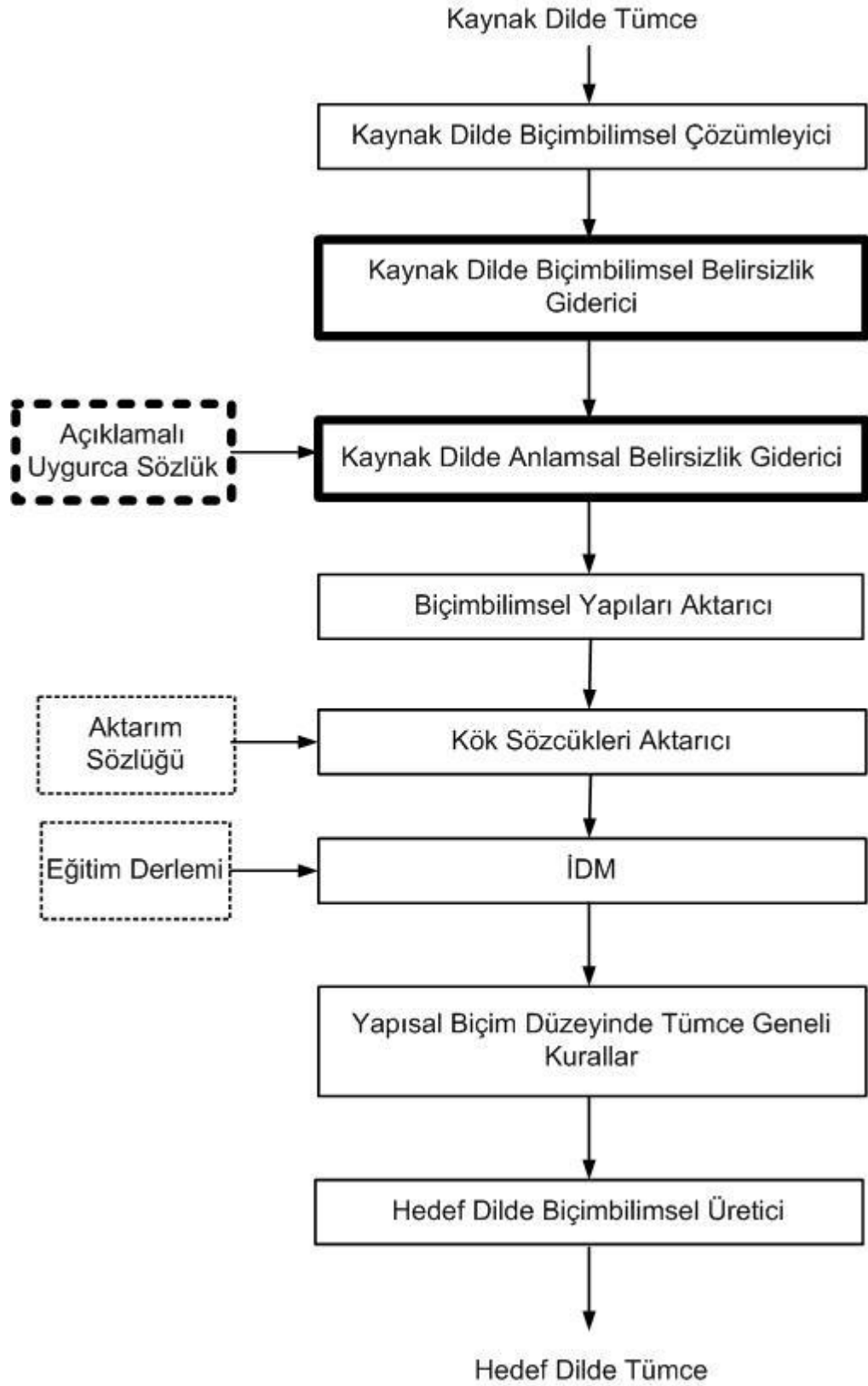
Şekil 6.3 : Belirsizlik giderme yöntemi([55]'den geliştirilmiştir).
