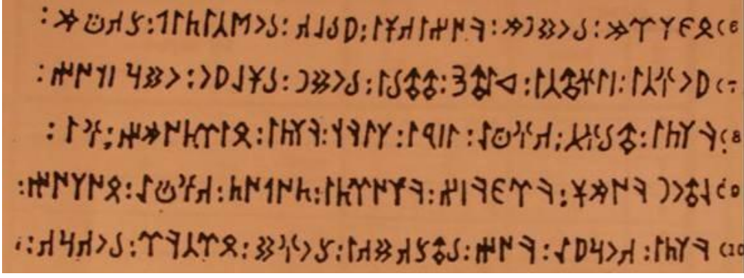
Şekil 3.1 : Orhun-Yenisey yazıtları [58].
