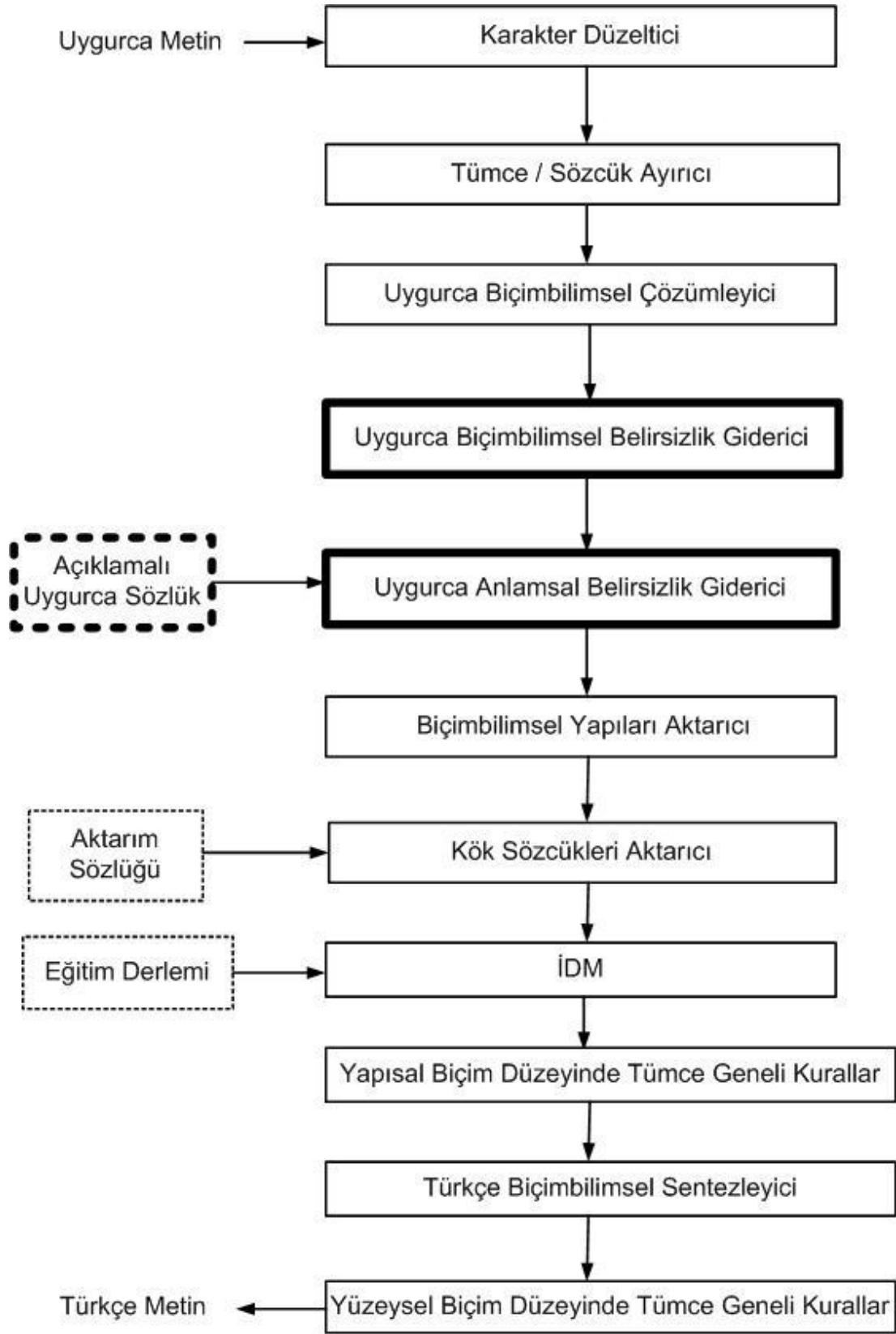
Şekil 7.2 : Belirsizlik giderme yöntemi ile çeviri sistemi
