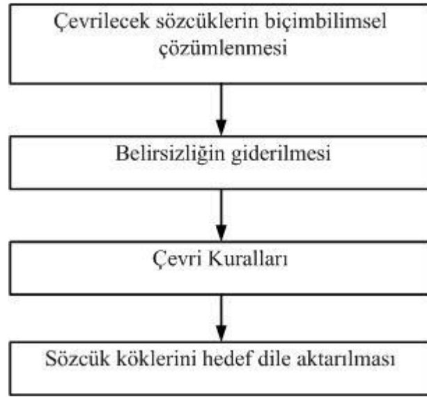
Şekil 2.2 : Yakın diller arasında bilgisayarlı çeviri aşamaları[52].
