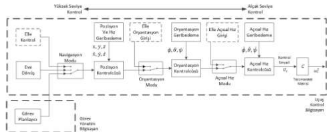
Şekil 2: Tam otonom hava aracının kontrol sistemi
