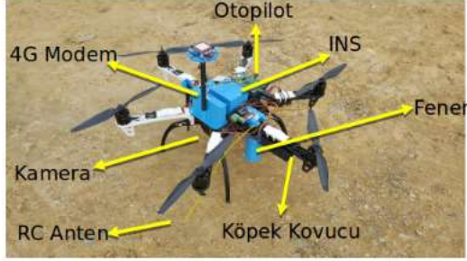
Şekil 1: Hava aracının genel görünümü.
