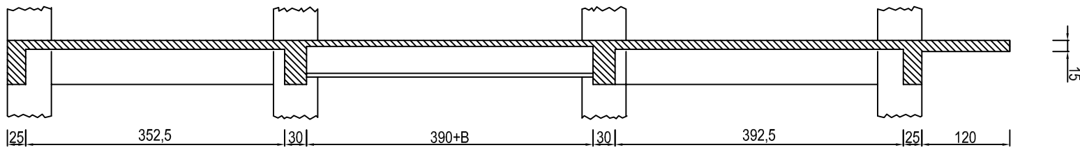
KESİT 3-3
