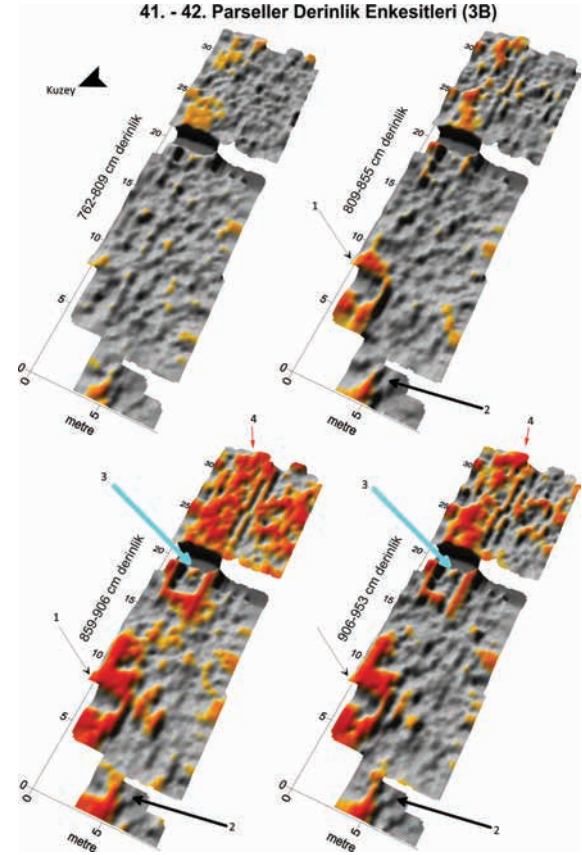
Şekil 21: 41 ve 42. parsellerdeki ölçüm sonuçlarına ait 3B açılı derinlik enkesitleri.
