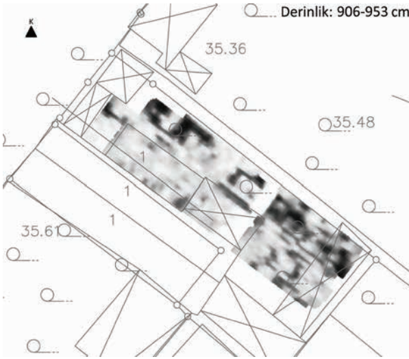
Şekil 20: Sultan Ahmet Camii 41 ve 42. parsellerdeki ölçüm sonuçlarının plan üzerine süperpozisyonuna bir örnek enkesit.
