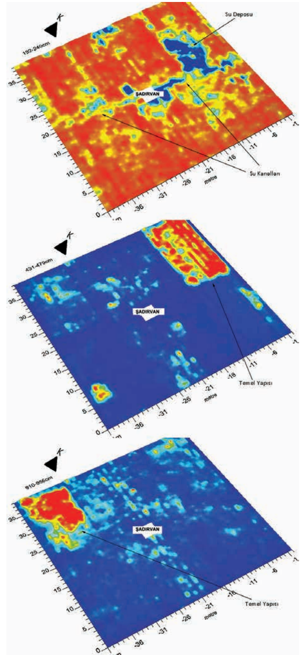
Şekil 8: İç Avlu alanına ait derinlik enkesitleri. Ortadaki boşluk avlu şadırvanına denk gelmektedir.
