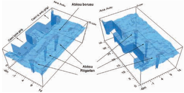
Şekil 12: Sultan Ahmet Camii içi jeoradar profillerinin oturumunu gösteren plan.
