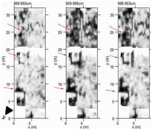
Şekil 19: 41 ve 42. parsellerdeki ölçüm sonuçlarına ait derinlik enkesitleri
